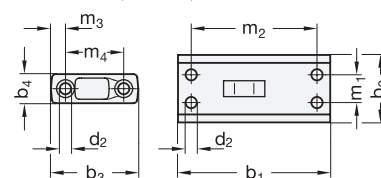
Anschlussmaße (Draufsicht)
