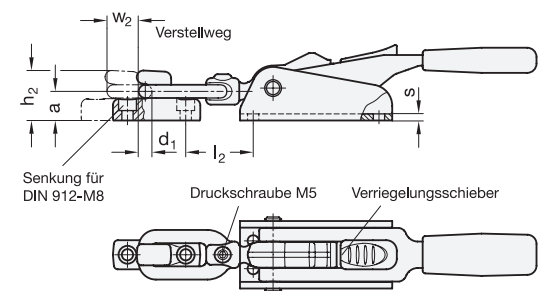
Anschlussmaße (Draufsicht)
